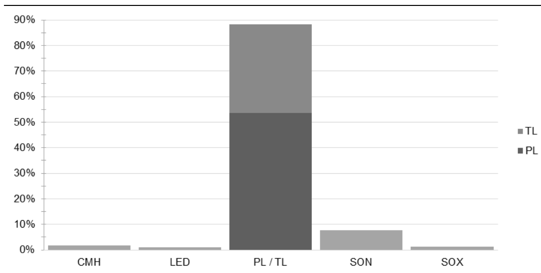
Figuur 3.4 Areaalopbouw van armaturen naar type lichtbron
