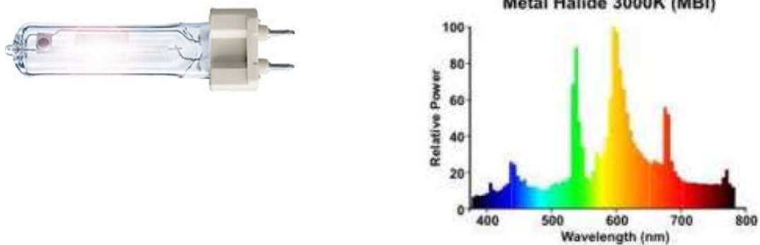
Figuur 4.1 Afbeelding CMH lichtbron en spectrale verdeling
