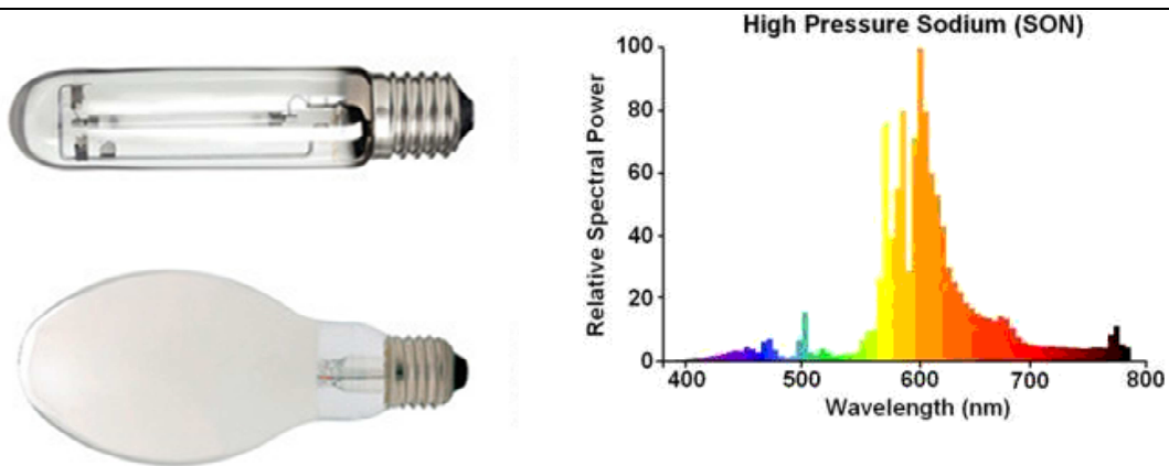
Figuur 2.1 Afbeelding SON lichtbron en spectrale verdeling
